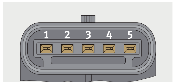
Belegung des Gehäusesteckers am AGR-Ventil
